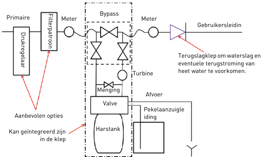
Blokschema
